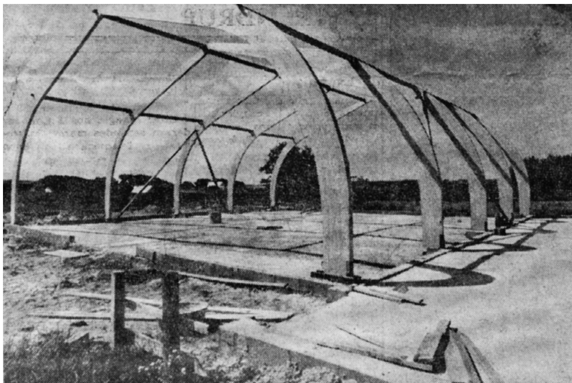
Støbearbejde er udført og buerne er rejst på den nye sognegård i Asdal. Efter sommerferien skal murerne i gang, og bygningen skulle stå færdig i løbet af efteråret.
